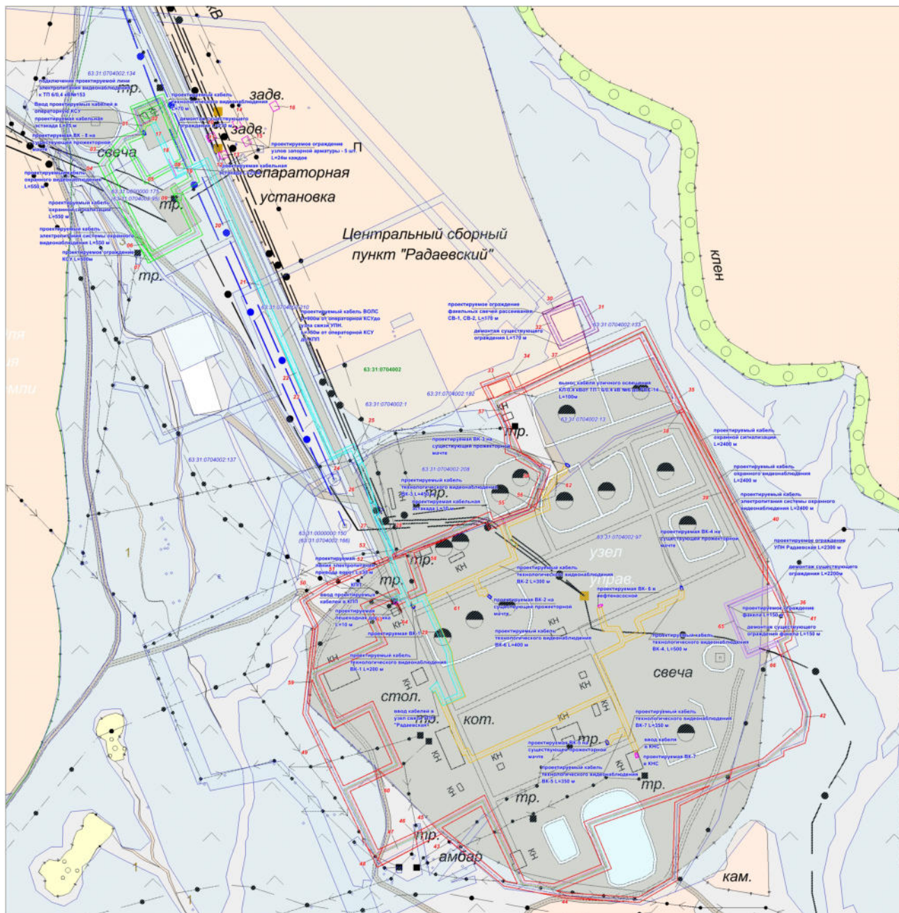
Масштаб 1:2 000
